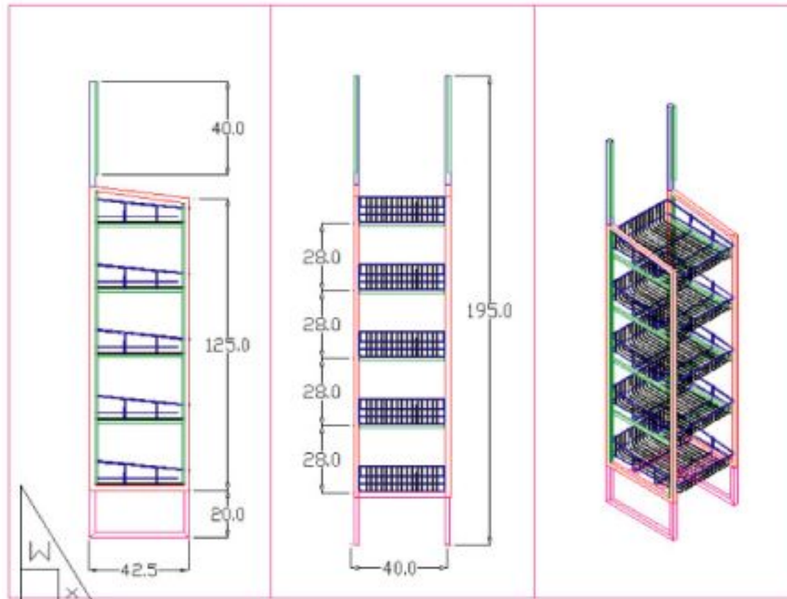
VISTA LATERAL
