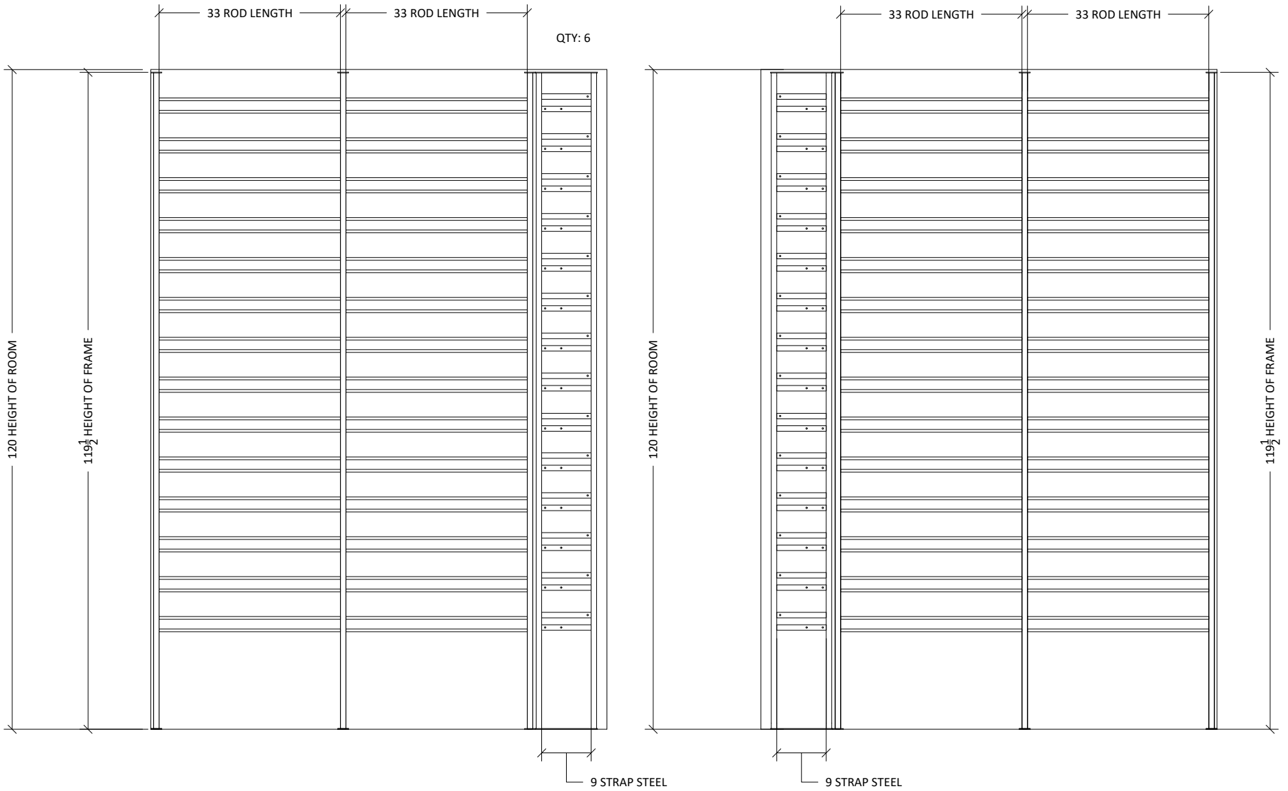
1 ELEVATION Scale: 1/2" = 1'-0"
