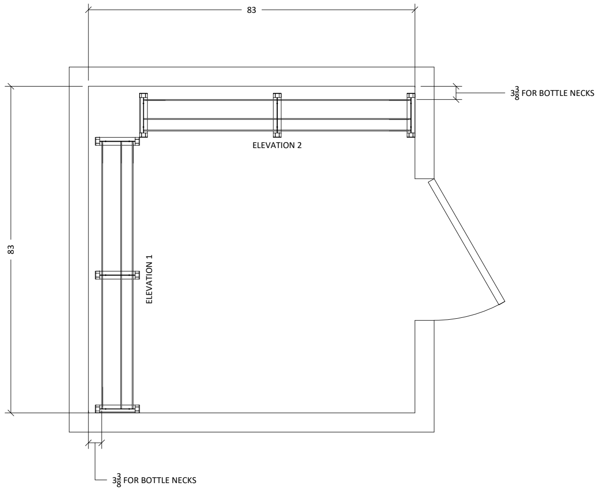
1 PLAN Scale: 1'0" = 1'-0"
