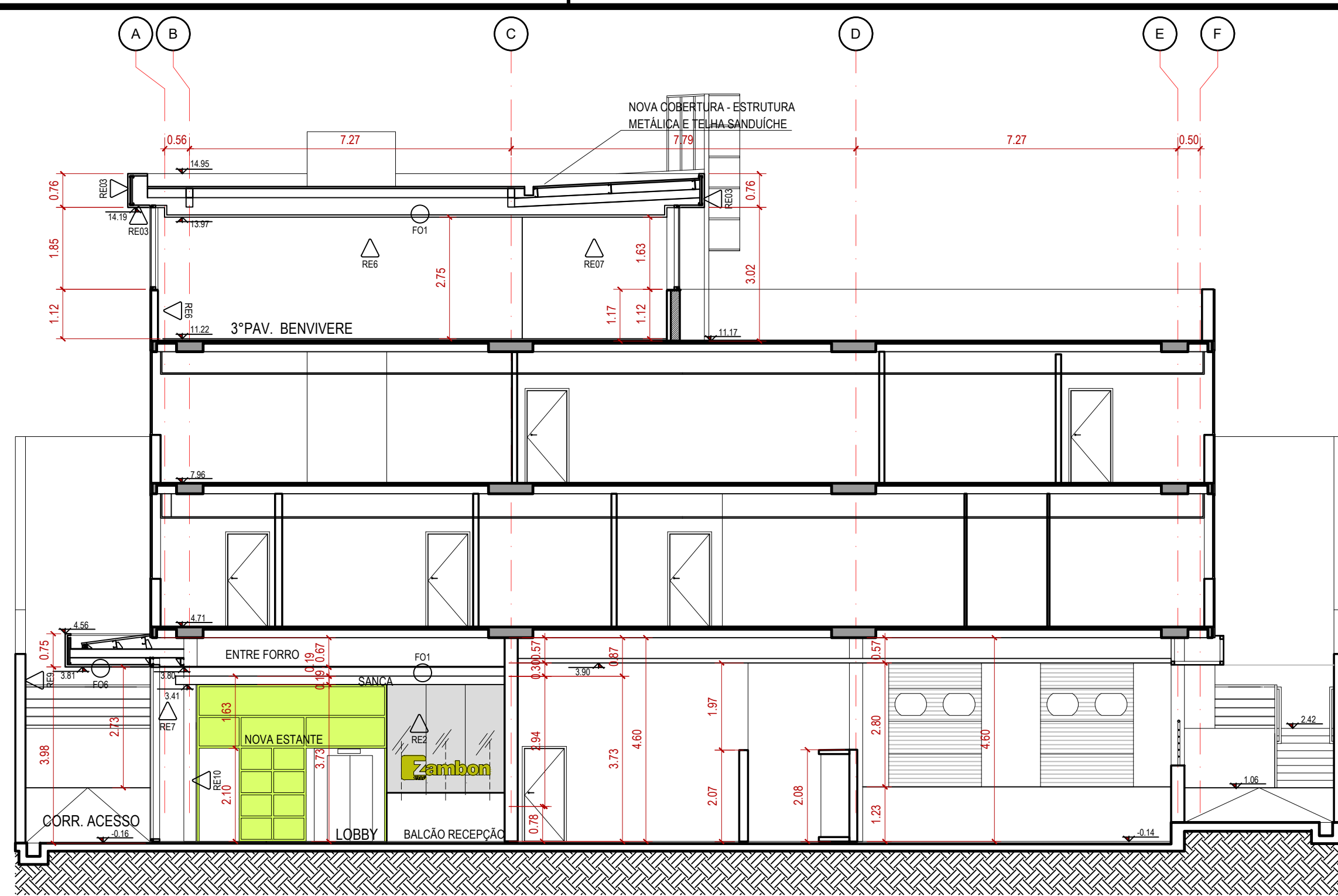
A CORTE A CORTE TRANSVERSAL ESCALA 1:100
