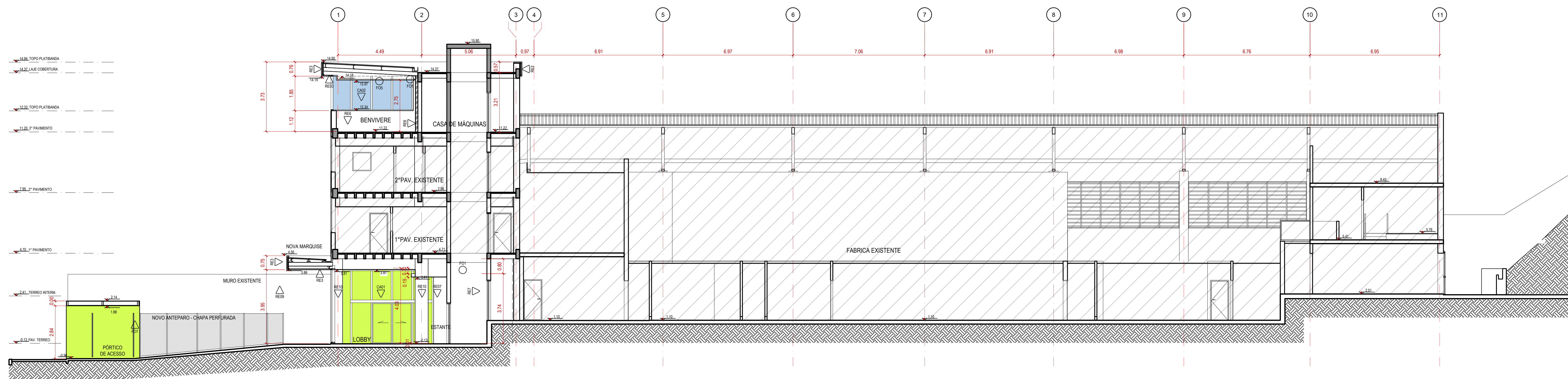
B CORTE B CORTE LONGITUDINAL ESCALA 1:100
