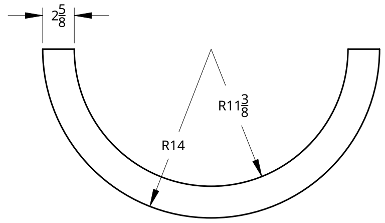
TRF-02
