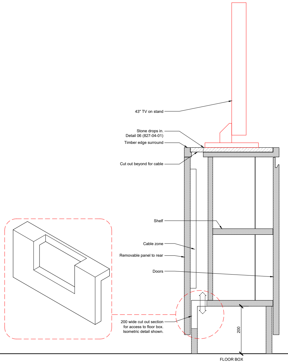
01 SECTION
