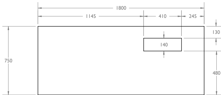
FLIPPER CUTOUT
