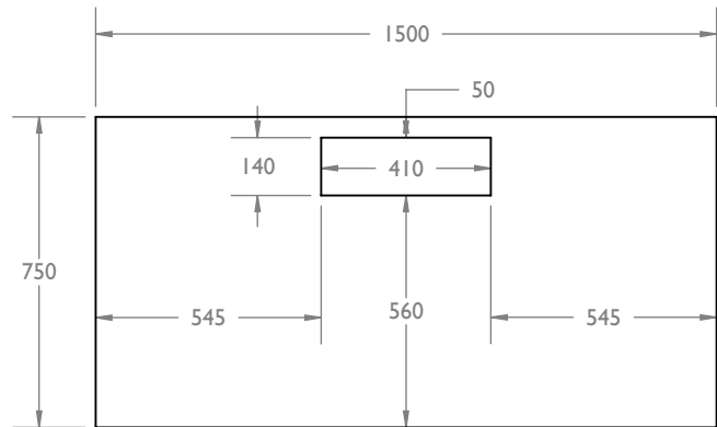
FLIPPER CUTOUT
