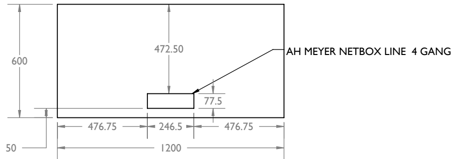
AH MEYER CUTOUT
