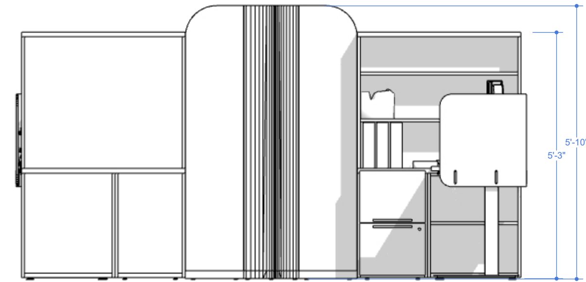
1 02 Elevation Scale: 1/4"=1'
