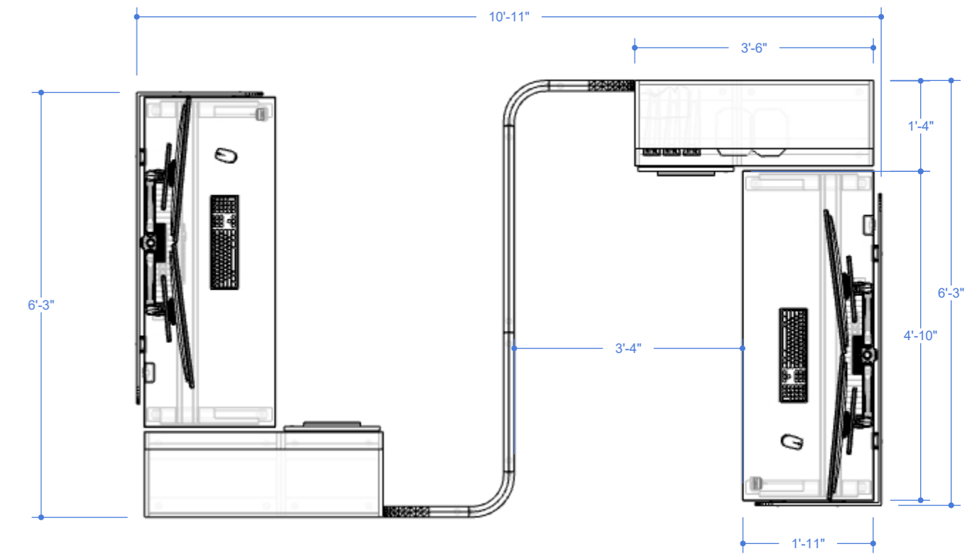
1 01 Plan Scale: 1/4"=1'
