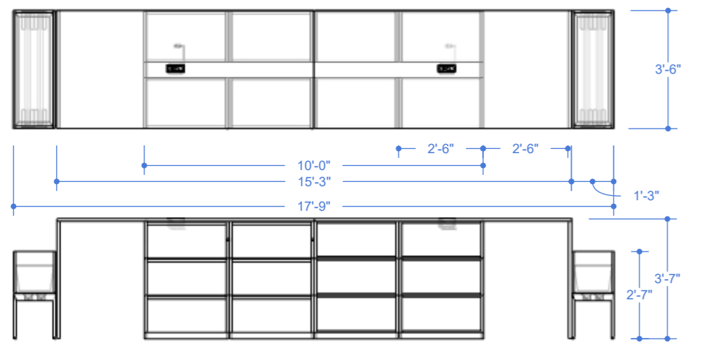
4 05 END-CAP TYPE E Scale: 1/4"=1'
